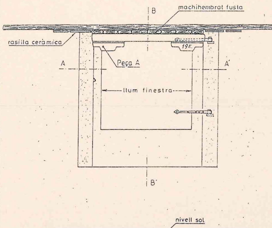
ALÇAT INTERIOR e. 1/20
