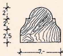
Detall A. (Pasamà) Secció A-A' e: 1/4
