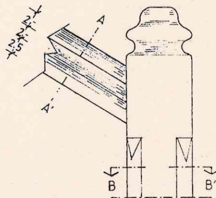
Detall B. e: 1/5
