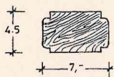
Detall D. Secció D-D' e: 1/4 cotes en cms.
