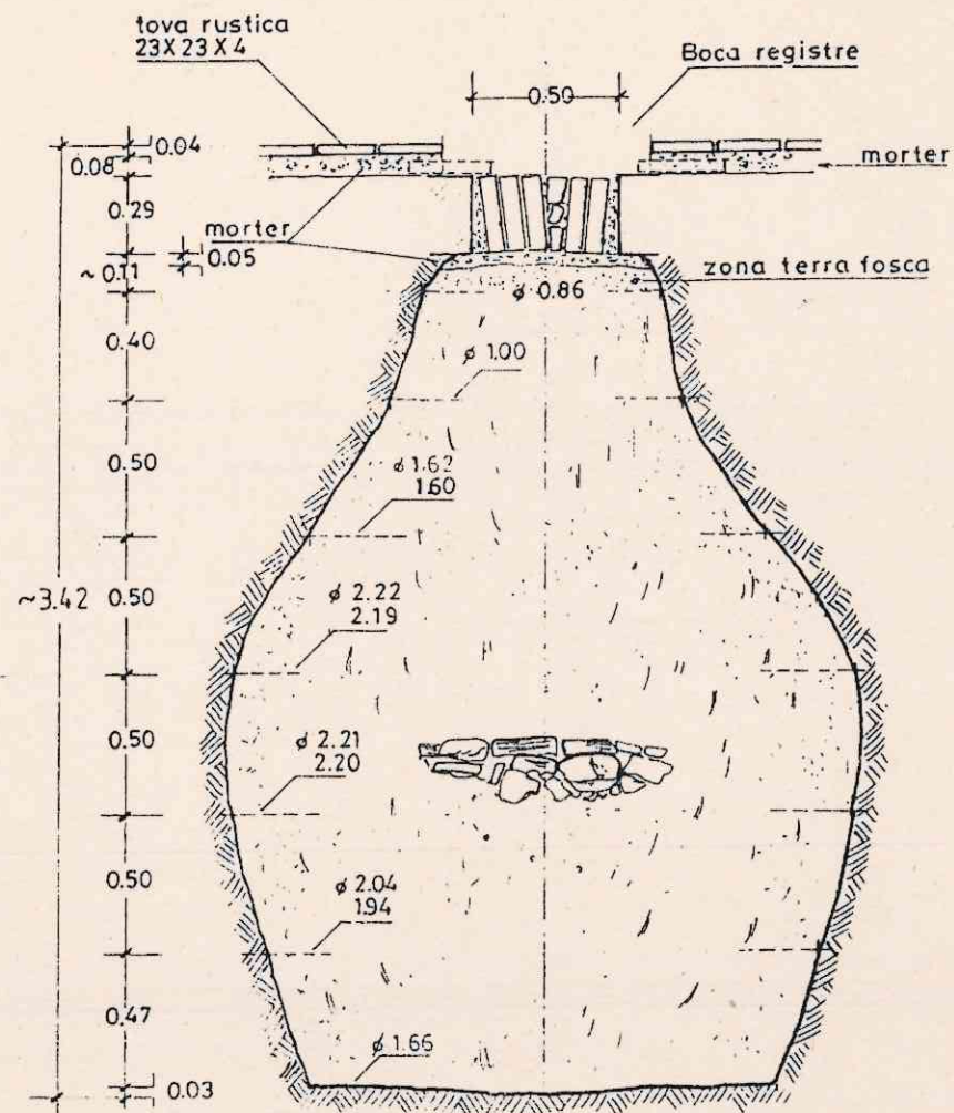
SECCIÓ A-A'
