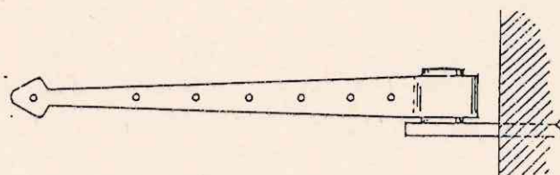
Detall frontissa porticó e. 1/5
